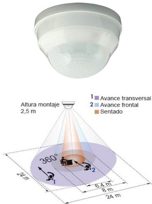
LUXOMAT®PD4
